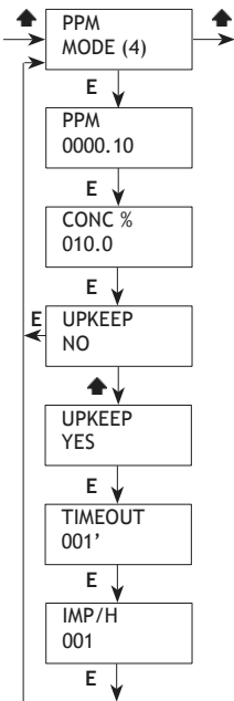
Fig. 17. PPM menu.
