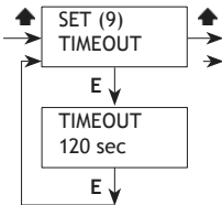
Fig. 37. Timeout menu.
