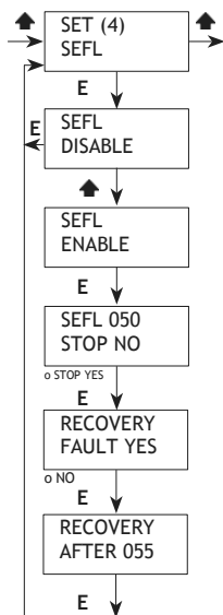
Fig. 32. SEFL menu
