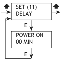
Fig. 40. Delay menu.
