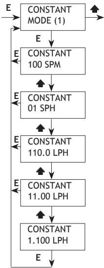
Fig. 14. Constant menu.
