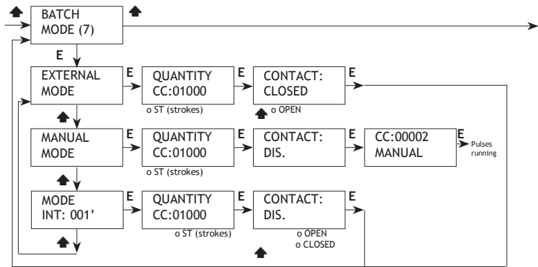
Fig. 20. BATCH menu
