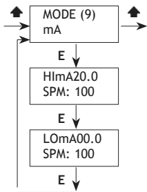
Fig. 24. mA mode
