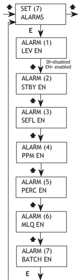
Fig. 35. Alarms menu.
