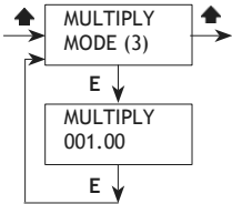
Fig. 16. Multiply menu.
