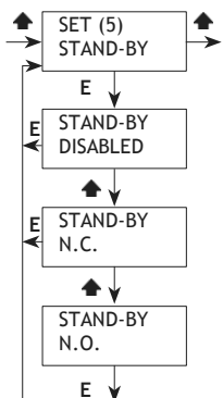
Fig. 33. Stand-by menu.
