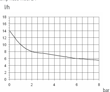
085,5: l/h 5,5 bar 8 Pump head mod. LA
