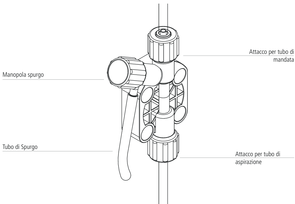
Fig. 6. Descrizione corpo pompa con spurgo manuale (VMS MF).
