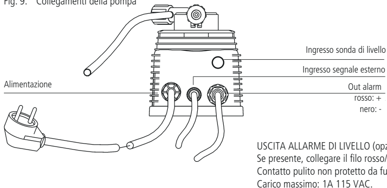
Fig. 9. Collegamenti della pompa
