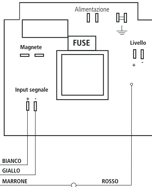
Fig. 39. Schema circuito VMS MF per la connessione ad un contatore lancia impulsi con effetto Hall
