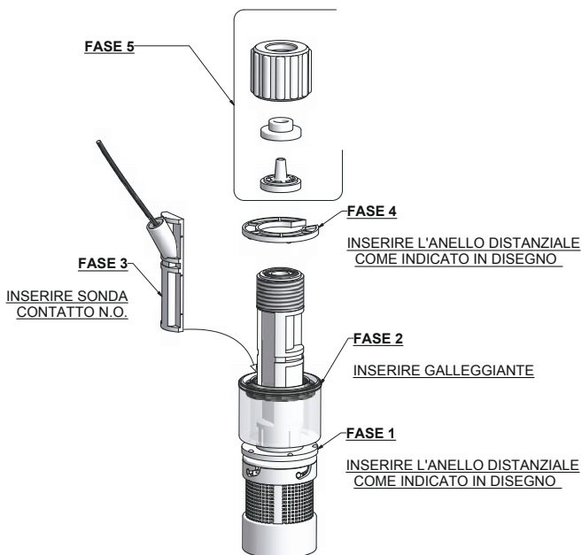
Fig. 3. Assemblaggio filtro di fondo / sonda di livell
