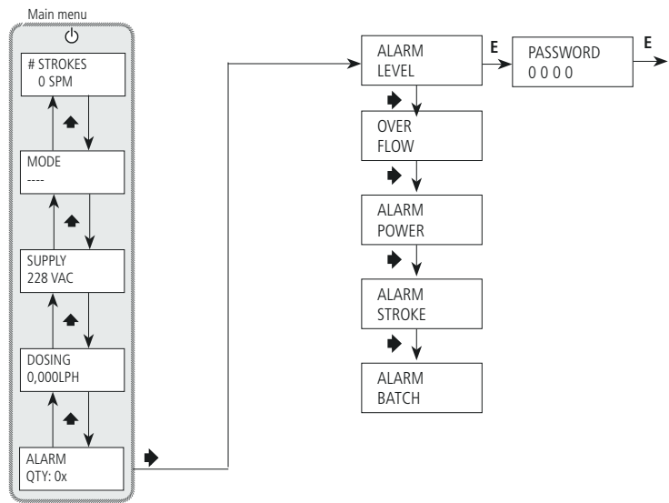
Fig. 37. Menù allarmi attivi.
