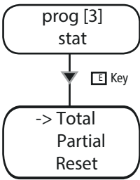
Fig. 36. Menù di gestione delle statistiche.
