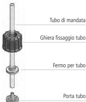
Fig. 4. Assemblaggio tubo mandata / corpo pompa
