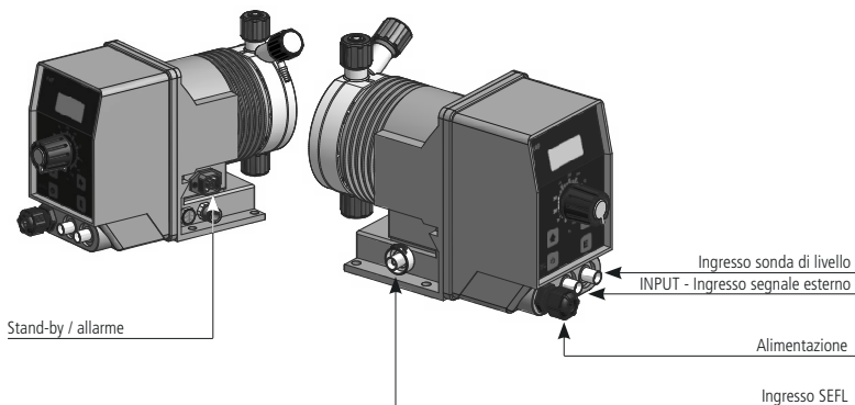
Fig. 12. Collegamenti della pompa
