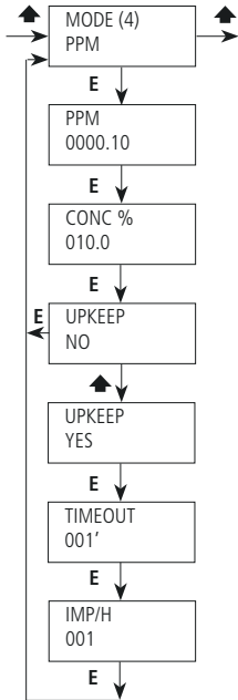
Fig. 17. Menù PPM.
