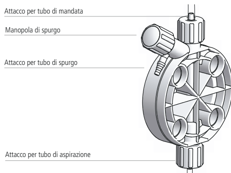
Fig. 7. Descrizione corpo pompa in PMMA con spurgo manuale (KMS MF).
