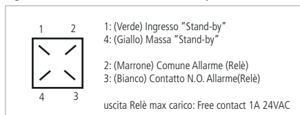
Fig. 11. Connessione allarme/stand-by
