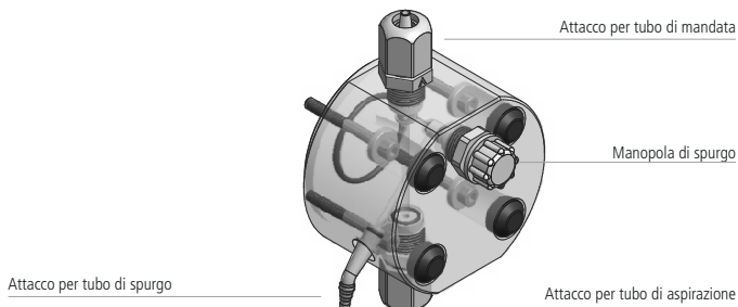
Fig. 7. Descrizione corpo pompa in PMMA con spurgo manuale (KMS MF).
