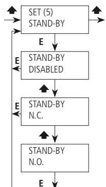
Fig. 33. Menù Stand-by.
