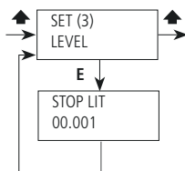
Fig. 30. Menù LEVEL
