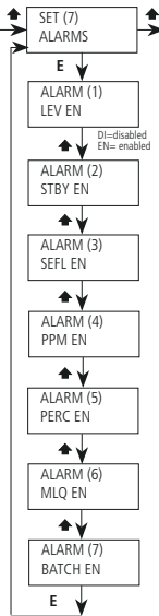
Fig. 35. Menù Alarms.
