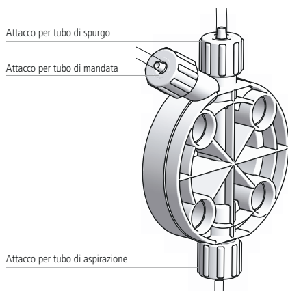
Fig. 8. Descrizione corpo pompa autospurgo (pompa KMSA MF).
