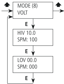
Fig. 26. Menù VOLT
