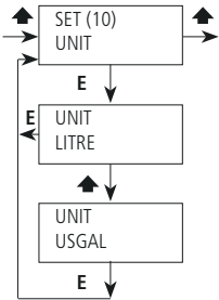
Fig. 39. Menù Unit.
