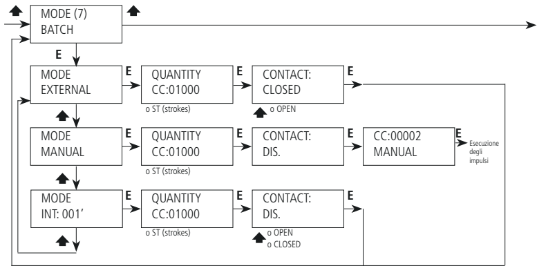
Fig. 20. Menù BATCH
