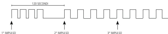
Fig. 38. Timeout.
