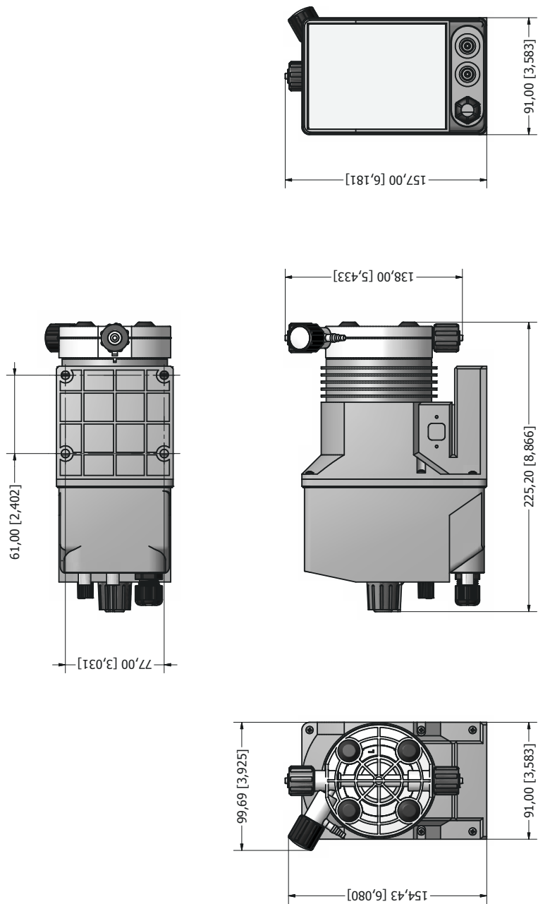
Fig. 48. Dimensioni pompa
