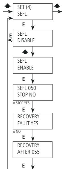
Fig. 32. Menù SEFL
