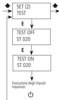
Fig. 29. Menù TEST
