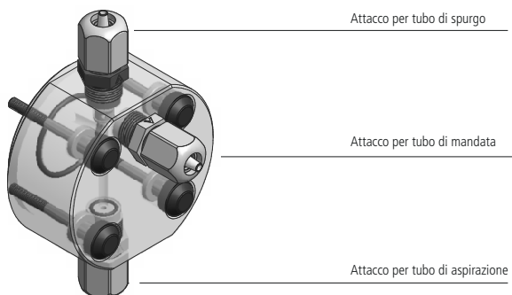
Fig. 9. Descrizione corpo pompa in PMMA autospurgo (pompa KMSA MF).
