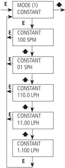
Fig. 14. Menù Constant.
