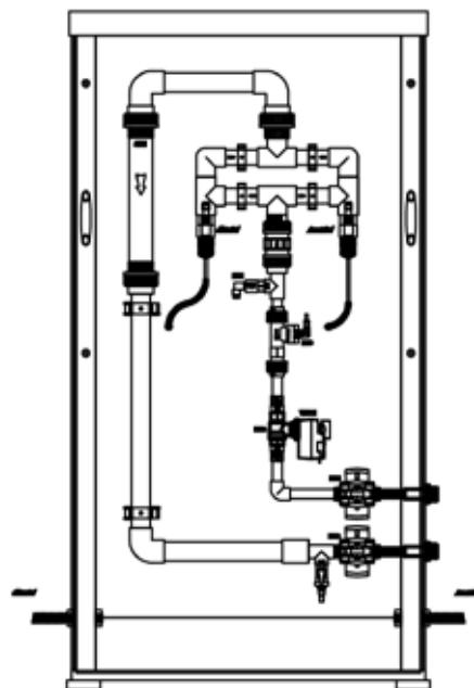
Fig. 2 - Pannello strumentazione (retro)
