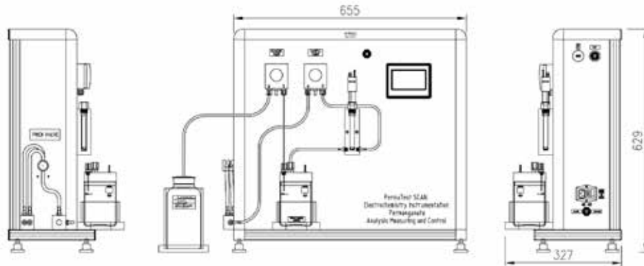
Fig. 1 - Pannello strumentazione
