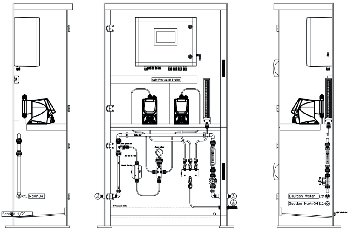
Fig. 1 - Pannello strumentazione
