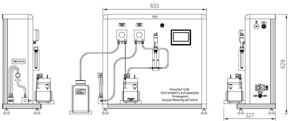
Fig. 1 - Pannello strumentazione
