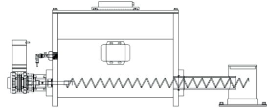
Fig. 2 - Tornillo de alimentación
