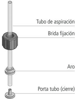
Fig. 3. Montaje tubo de aspiración / filtro de fondo
