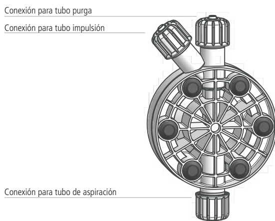
Fig. 7. Cabezal autopurgante mod.: SA, TA (bomba TA).
