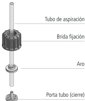
Fig. 4. Montaje tubo de impulsión / cuerpo de bomba
