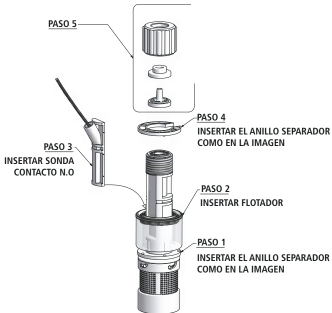
Fig. 2. Montaje filtro de fondo / sonda de nivel
