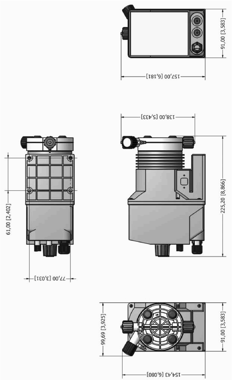
Fig. 49. Dimensiones bomba
