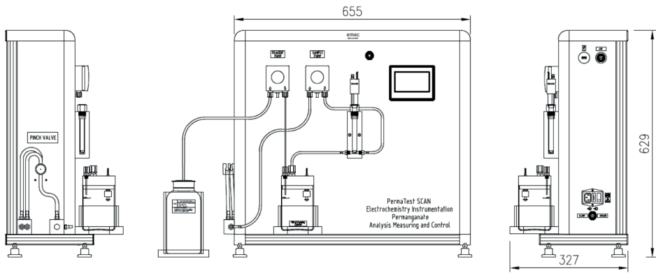
Fig. 1 - Panel de instrumentación
