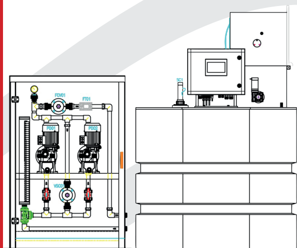
Fig. 2 - Esquema PermaDos SE + Skid Safety Box
