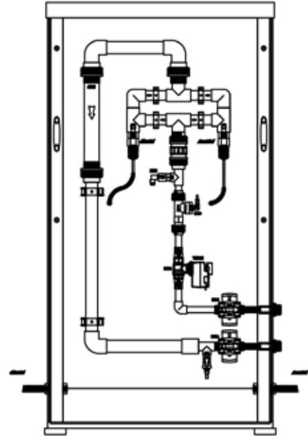
Abb. 2 - Aufbau (Rückseite)
