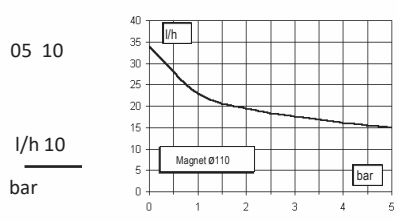
Pumpenkörper LA
