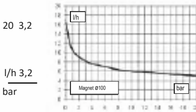
Pumpenkörper LA
