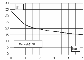
Pumpenkörper L
