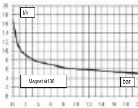
Pumpenkörper L
