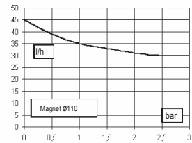
Pumpenkörper S
