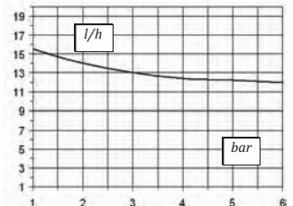
Einzeleinspritzung 1,66
